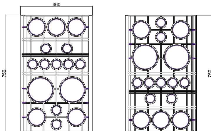
CAIXA PP 400X400X750
